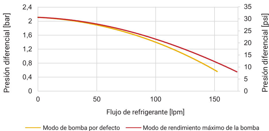
Curva P-Q secundaria (agua) con conexión Tri-Clamp
