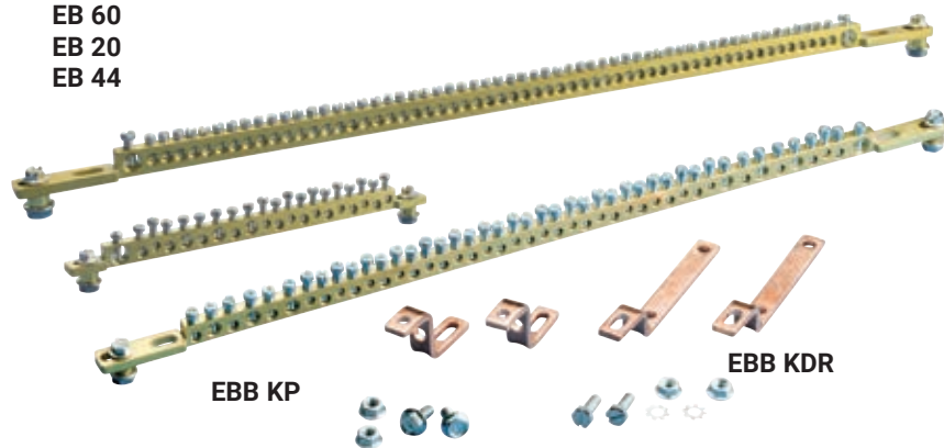
Montage sur barre cuivre
